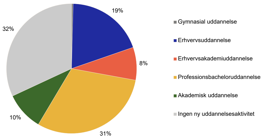
Figur 11. Ny uddannelsesaktivitet blandt frafaldne fra socialrådgiveruddannelsen 2010-2020
